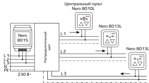
Рис. 1 — Схема передачи сигнала управления (технология PLC)
